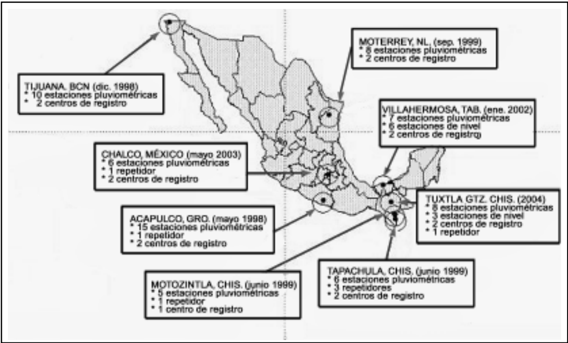
Fig. 53. Ubicación de los sistema de alerta hidrometeorológica instalados hasta 2004.
